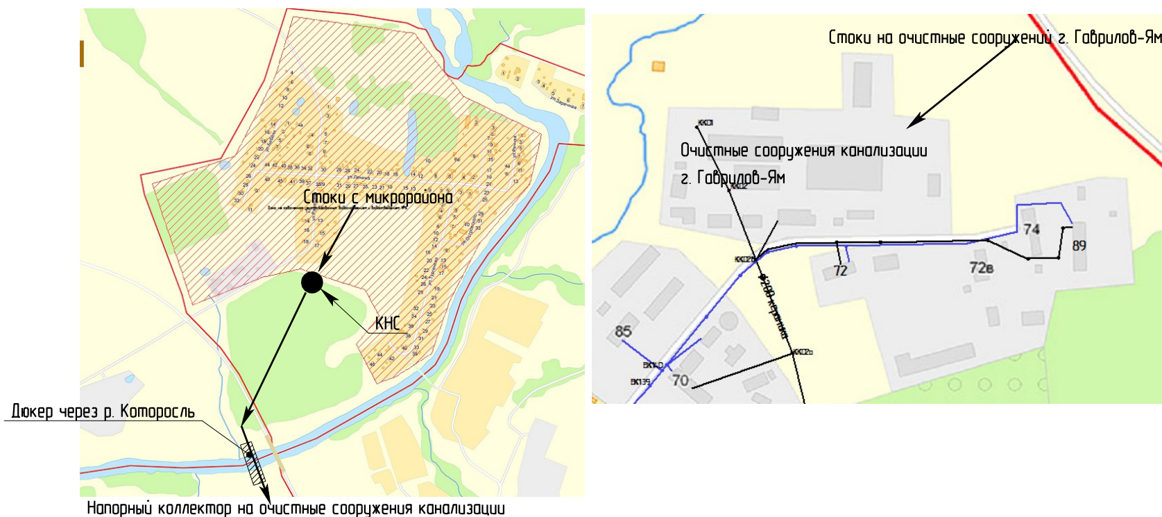
Рисунок 4.5 – Приблизительная схема подключения микрорайона к сетям водоснабжения
