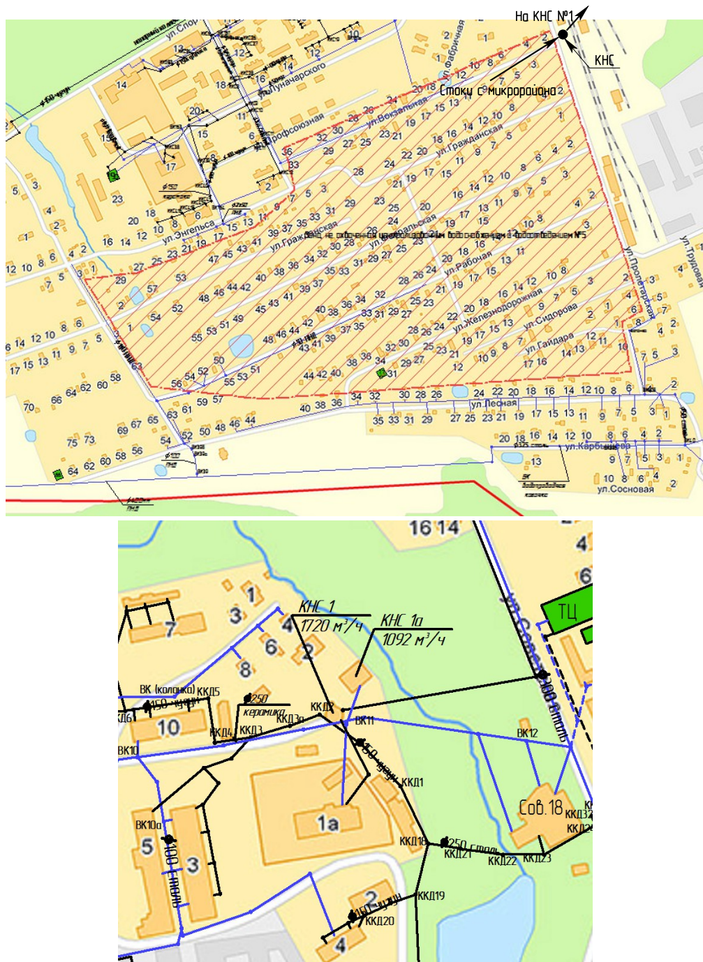
Рисунок 4.4 – Приблизительная схема подключения микрорайона к сетям водоснабжения
